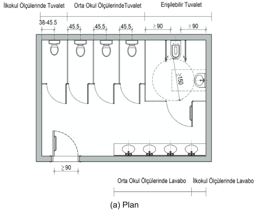
Şekil 6.7. Ortaokul ve Lise Tuvaleti
