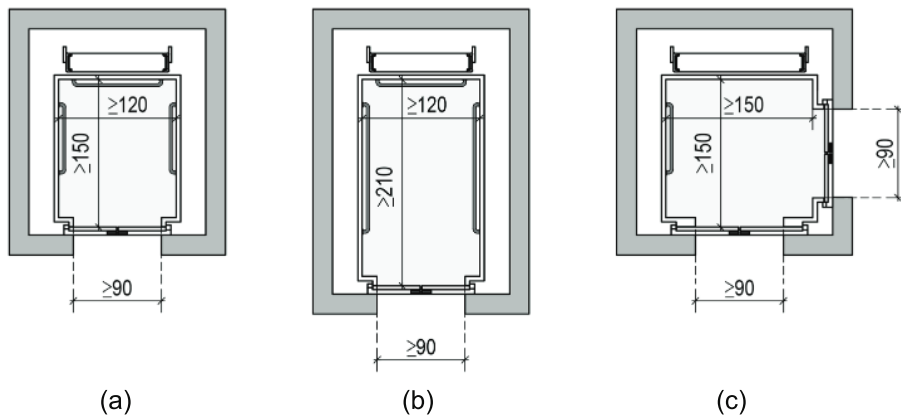
Şekil 8.1. Kabin Ölçüleri
