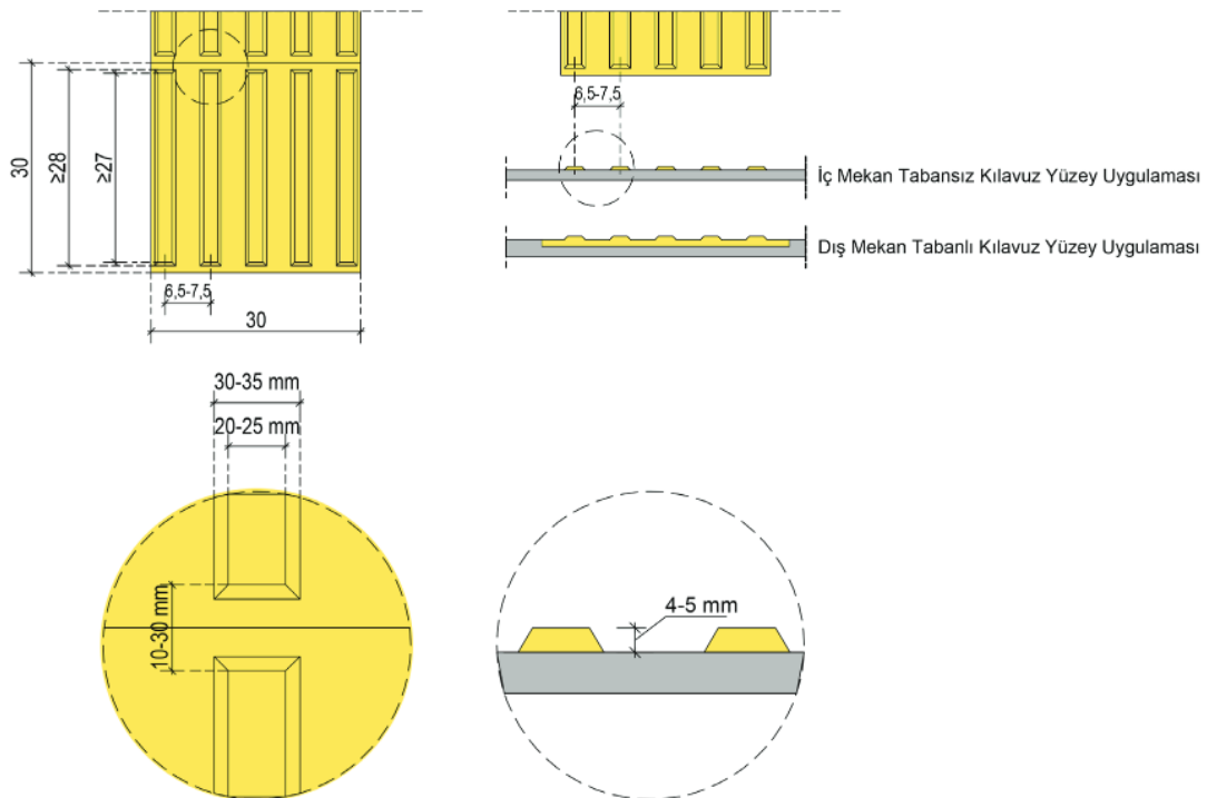
Şekil 11.1. Kılavuz Yüzey
