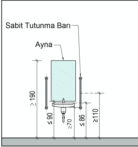
Şekil 6.20. Tutunma Çubukları
