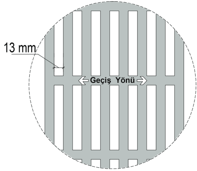
Şekil 1.17. Izgara Aralıkları
