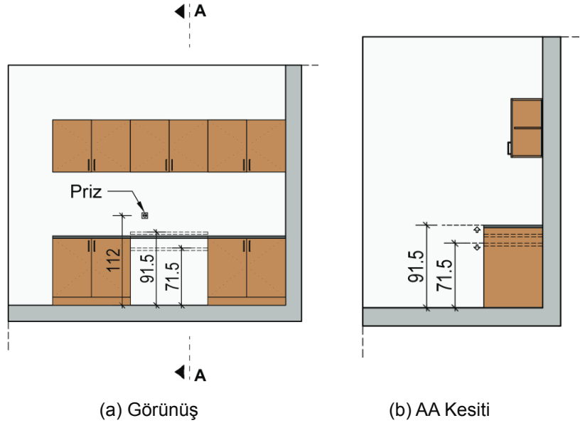
Şekil 12.1.3. Ayarlanabilen (Hareketli) Tezgâh Ölçüleri
