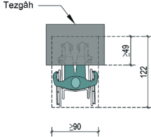
Şekil 12.1.2. Mutfaktaki Tezgâh Ölçüleri
