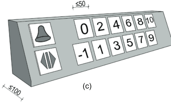
Şekil 8.5. Yatay Kontrol Paneli (Ölçüler mm'dir.)
