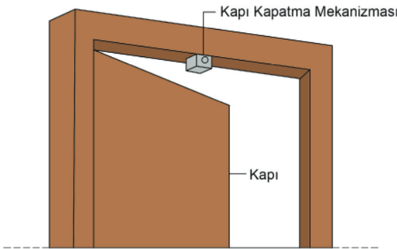
Şekil 5.13. Kapı Kapatma Mekanizması
