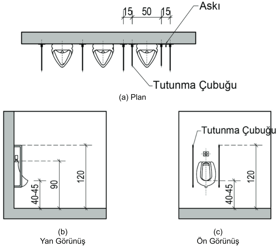
Şekil 6.18. Pisuvarlar
