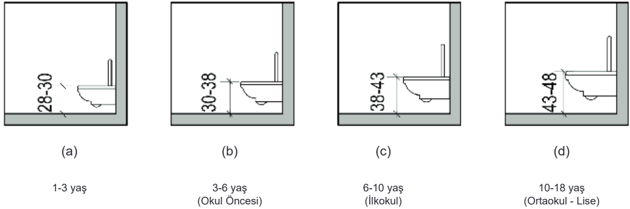
Şekil 6.8. Yaş Gruplarına Göre Klozet Kesitleri
