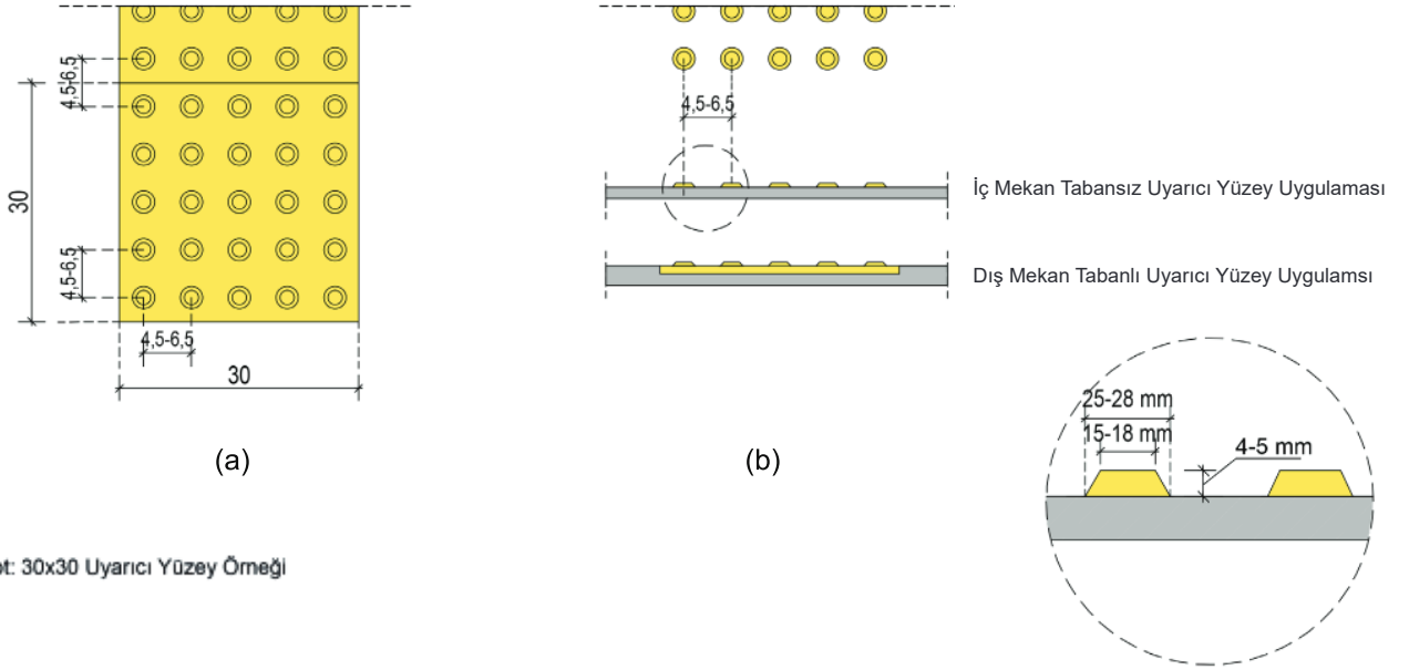
Şekil 11.2. Uyarıcı Yüzey
