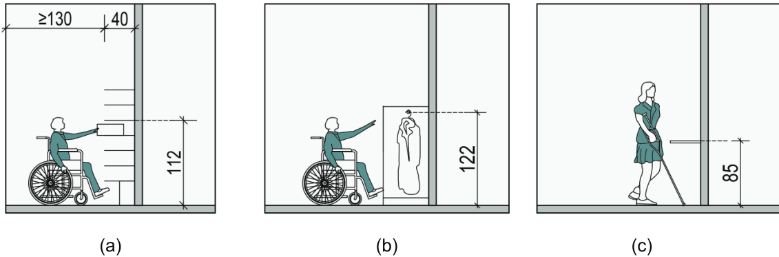
Şekil 1.14. Yandan Yaklaşım Mesafeleri
