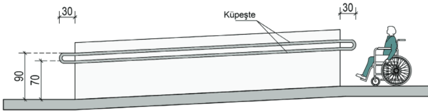
(b) Duvarda Küpeşte Uygulaması
