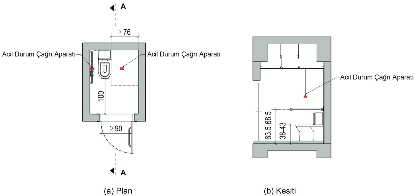
Şekil 6.9. Destekli Tuvalet Örneği
