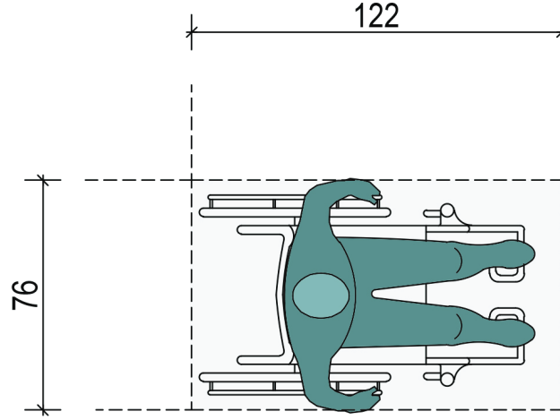
Şekil 1.3. Tekerlekli Sandalyenin Net Zemin veya Döşeme Alanı
