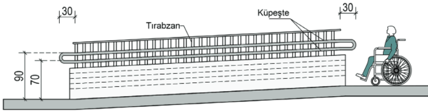
(c) Tırabzanlı Parapette Küpeşte Uygulaması
