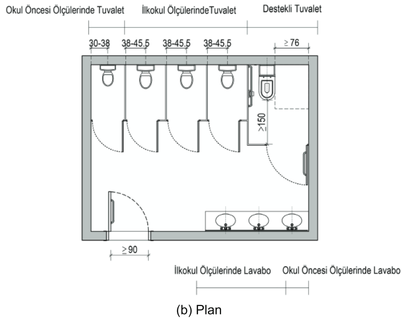
Şekil 6.6. İlkokul Tuvaleti
