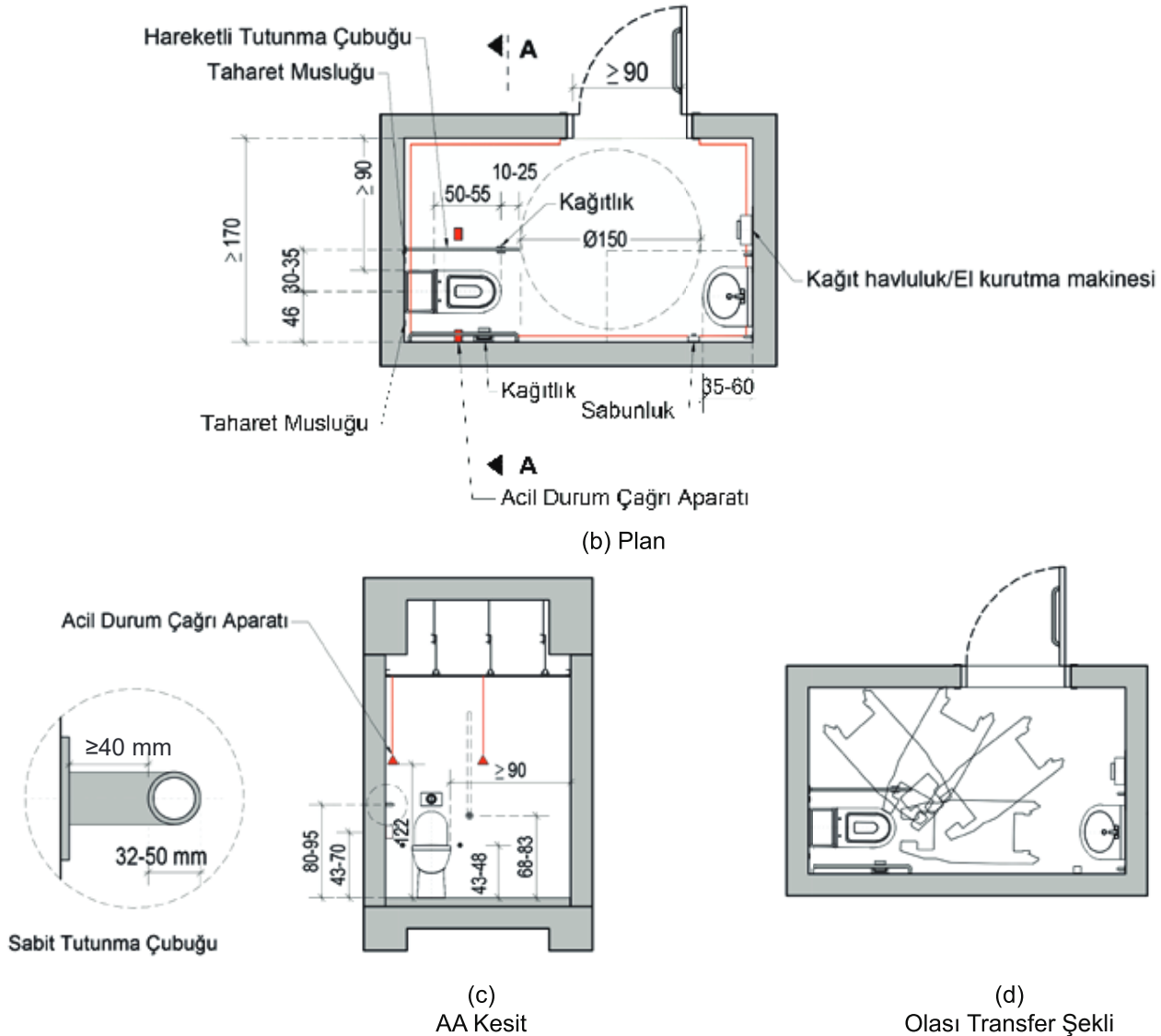
Şekil 6.2. Kapalı Alanı 800 m 2 Altı Binalarda Tuvalet Örneği
