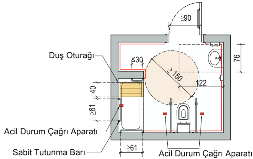
Şekil 12.2.4. Küvet ve Tuvaletin Birlikte Olduğu Banyo Örneği
