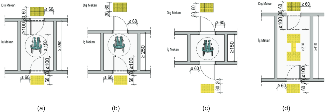
Şekil 4.8. Rüzgârlık Alanı ve Kapı Önlerindeki Uygun Manevra Alan Ölçüleri
