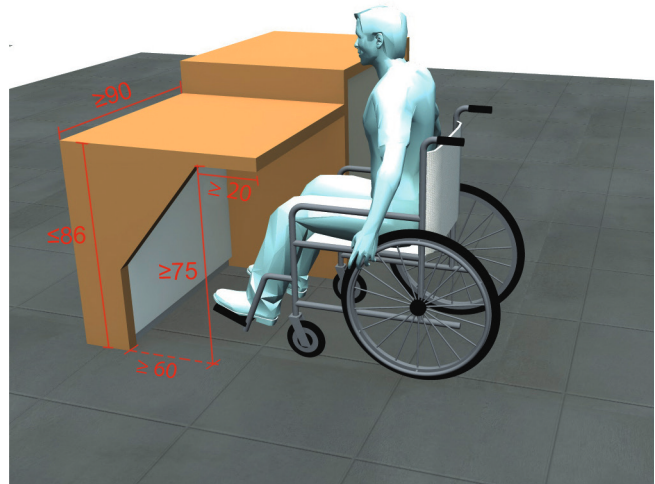
Şekil 4.12. Erişilebilir Banko
