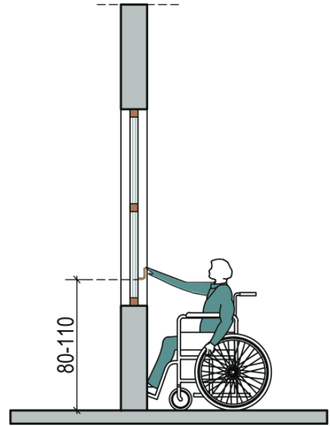
Şekil 5.14. Pencere Kolu Yüksekliği (Tekerlekli sandalye ile önden ve yandan yaklaşım için)
