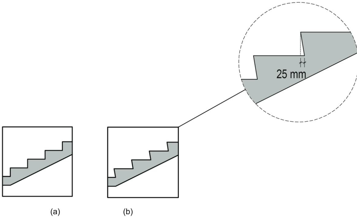
Şekil 1.27. Basamak Özellikleri
