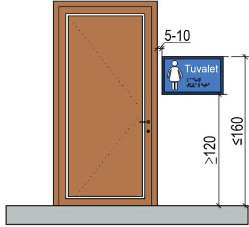
Şekil 10.2. Kapı Yanı İşaretlemeleri için Uygun Yükseklikler
