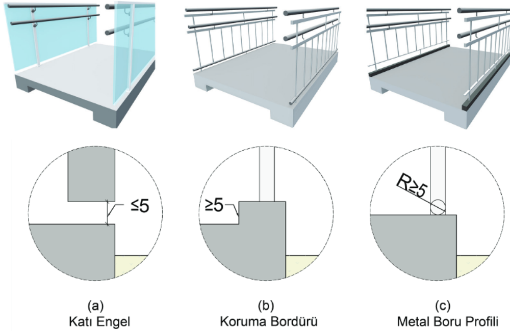
Şekil 1.24. Koruma Bordürü
