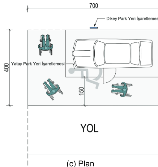
Şekil 3.1. Erişilebilir Park Yeri Tasarımı
