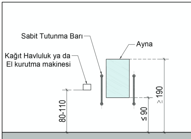
Şekil 6.21. Ayna
