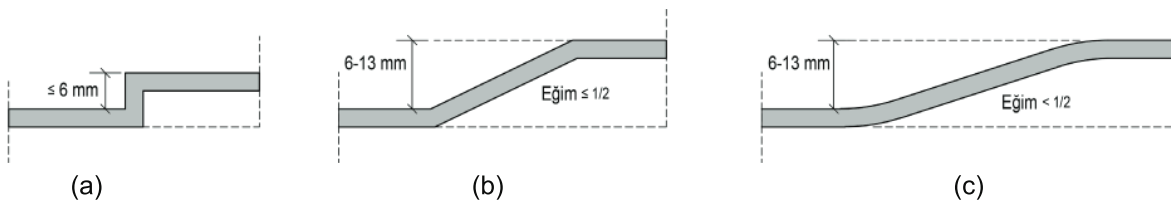
Şekil 1.16. “6 mm -13 mm” Arasındaki Seviye Farklılıkları İçin Düzenleme
