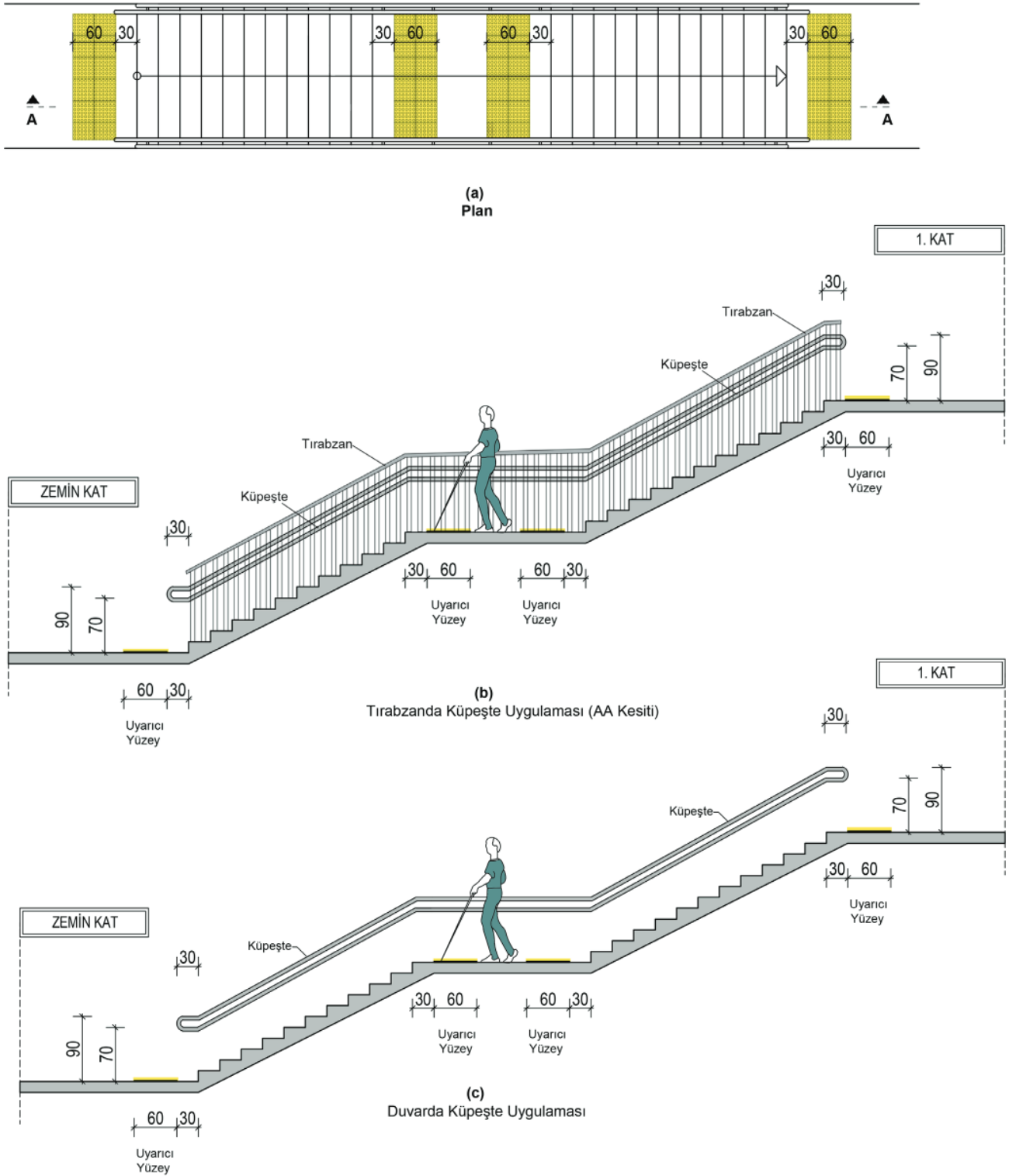
Şekil 1.26. Merdiven Ölçüleri
