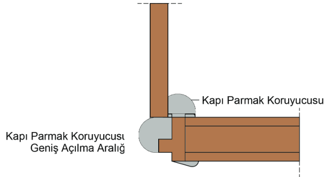
Şekil 5.12. Kapı Parmak Koruyucusu
