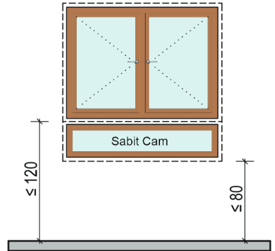
Şekil 5.15. Sabit Camlı Pencere Örneği
