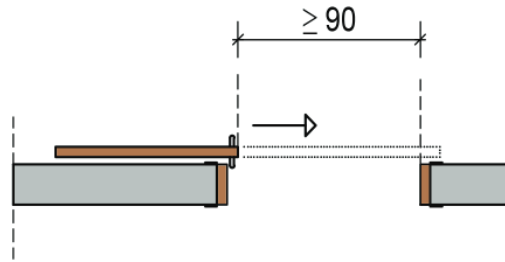
(b) Sürgülü Kayar Kapı
