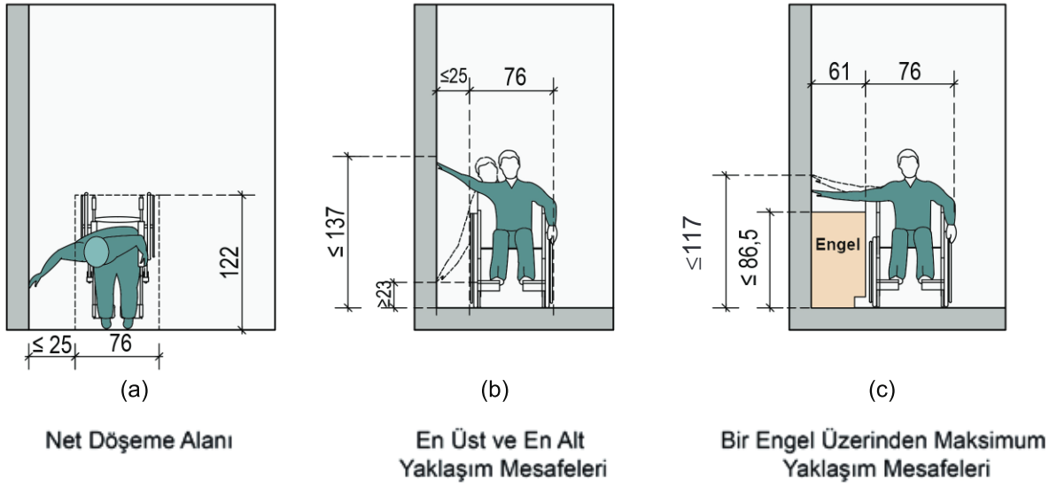
Şekil 1.13. Tekerlekli Sandalye İle Yandan Yaklaşım Mesafeleri
