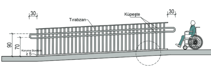
(a) Tırabzanda Küpeşte Uygulaması
