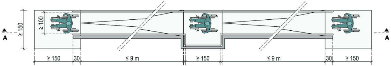
(a) Rampa Üstten Görünüş
