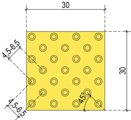
Şekil 11.3. Şaşırtmalı Uyarıcı Yüzey
