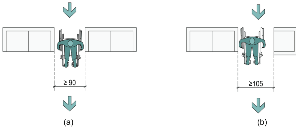
Şekil 12.3.3. Oturma Odası Geçiş Genişlikleri
