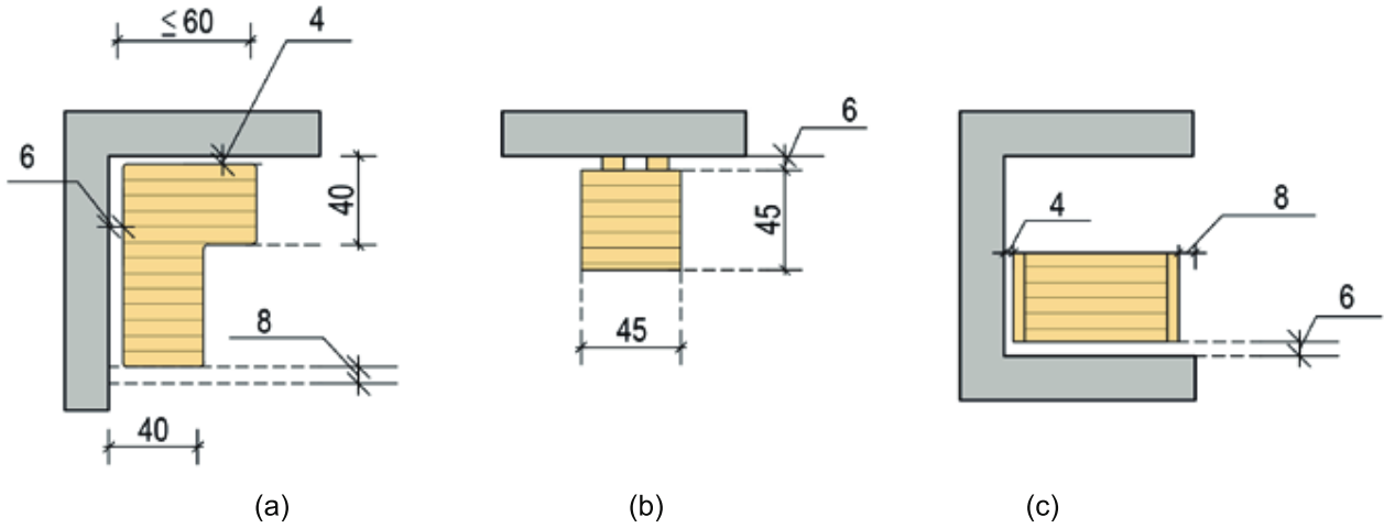
Şekil 12.2.8. Oturak Ölçüleri
