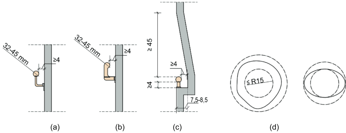
Şekil 1.23. Kúpeşte Örnekleri
