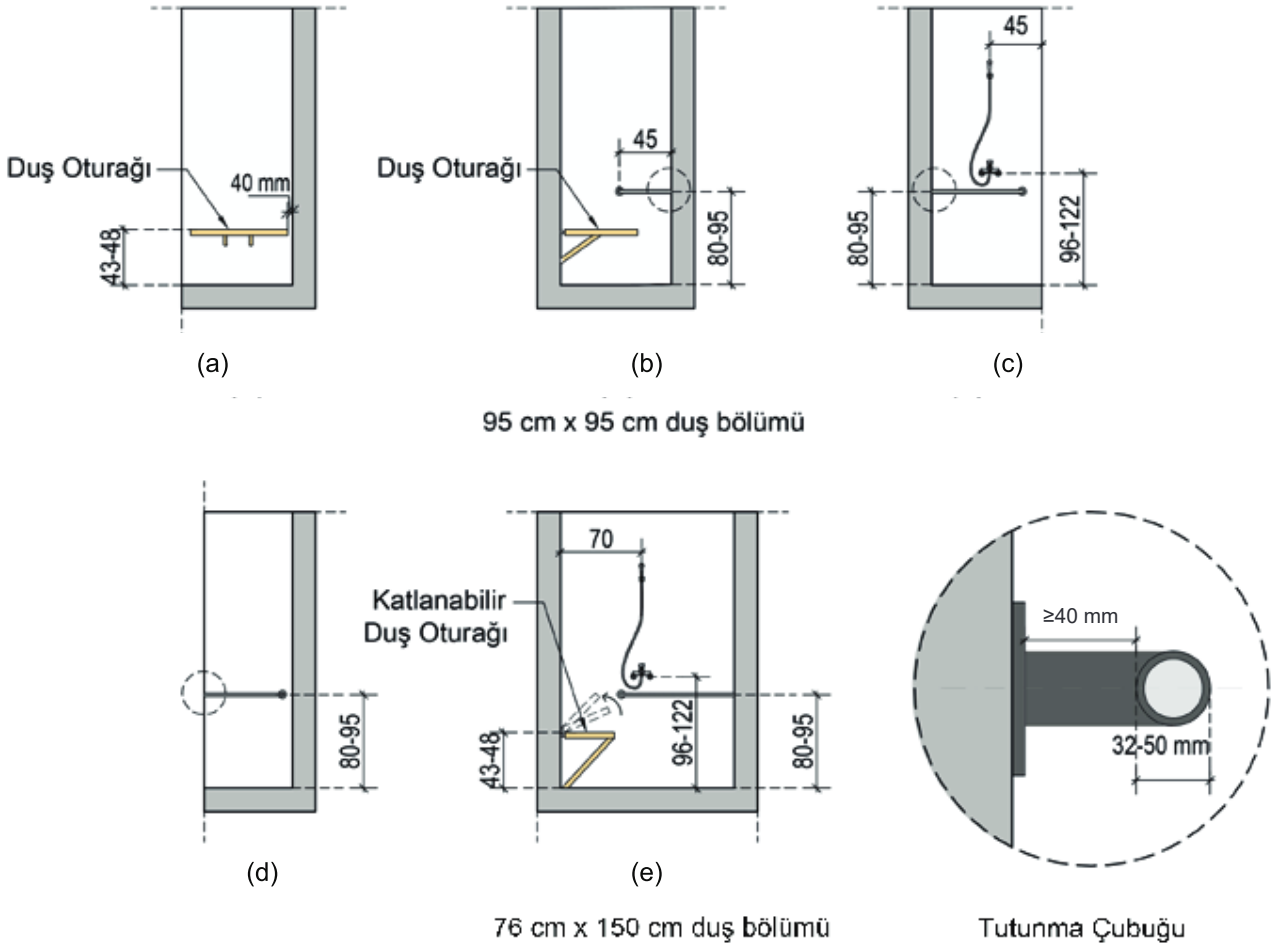
Şekil 12.2.7. Tutunma Çubukları, Su Kontrolü ve Oturak Ölçüleri
