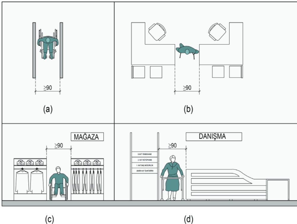
Şekil 1.2. Erişilebilir Güzergâh Genişliği
