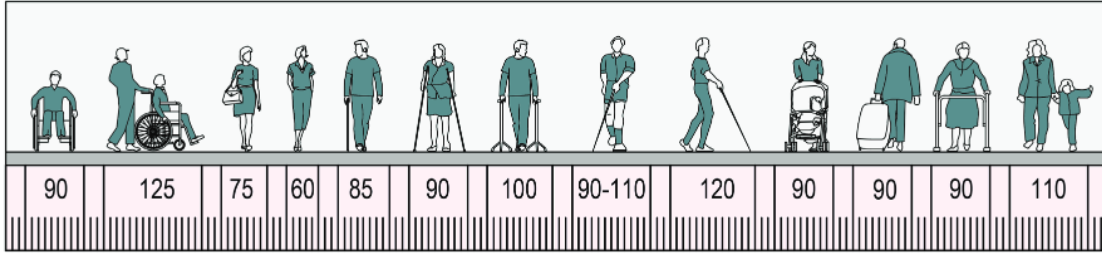
Şekil 1.1. Genel Ölçüler
