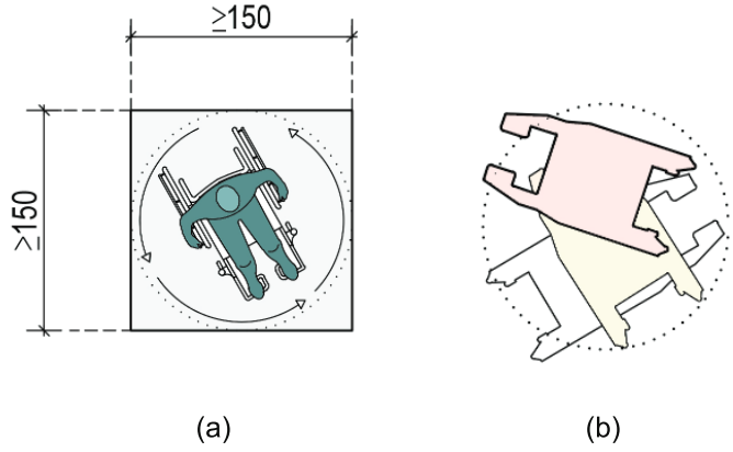
Şekil 1.7. Tekerlekli Sandalye Dönüş Alanları
