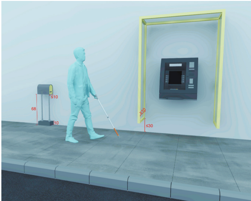
Şekil 2.4. Yaya Yürüyüş Alanında Engel Oluşturan Objelerin Konumlandırılması
