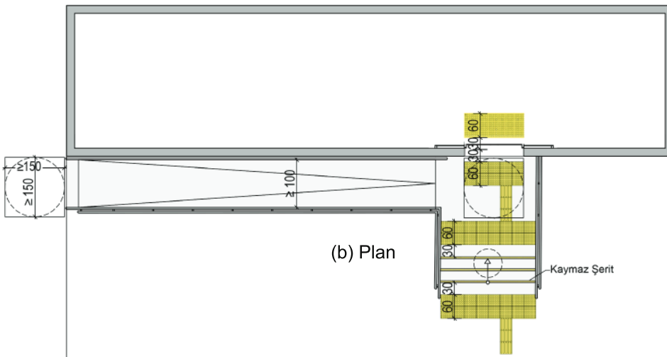
Şekil 4.1. Bina Girişi Düzenlemesi
